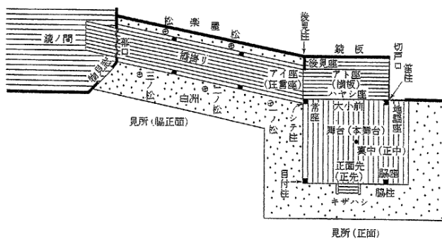
能舞台図
